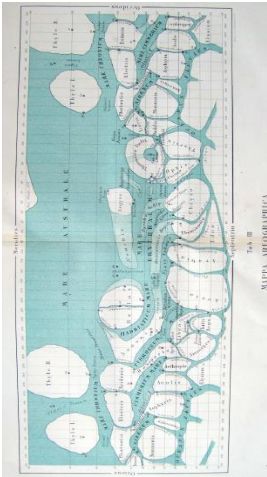
Tavola Mappa aerografica del pianeta Marte disegnata dall'astronomo, edita nella prima memoria lineica (cfr. Schiaparelli, Osservazioni astronomiche ... l'opposizione del 1877, 1878 cit., Tav. III ).
